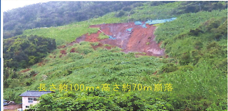
令和3年8月17日の国道路肩斜面崩落
